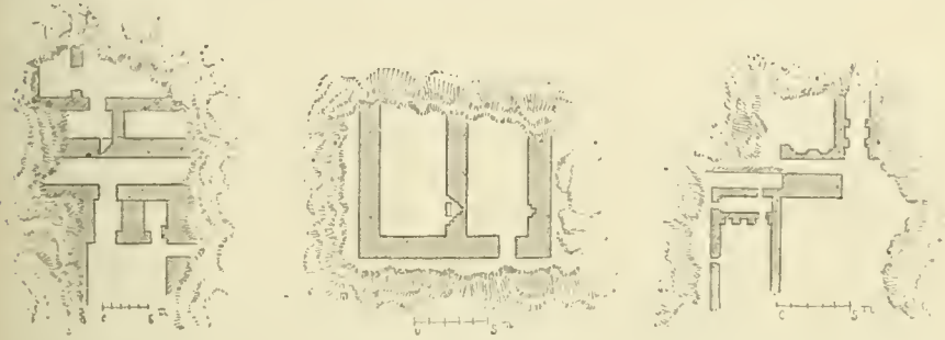
200. — Moughêir. Chambres. Plan, d'après Taylor. 201. — Abou-Shareïn. Chambres. Plan, d'après Taylor. 202. — Abou-Shareïn. Chambres. Plan, d'après Taylor.
